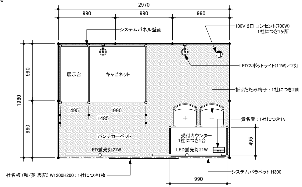
[平面図]
